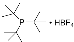
Tri-tert-butyl phosphine
