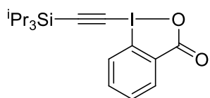
TIPS-EBX
